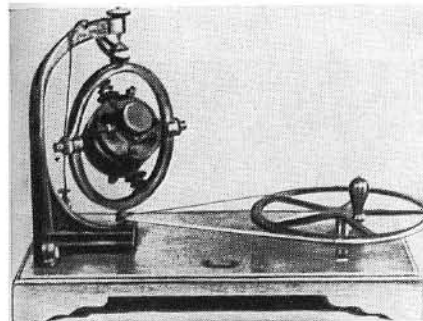
Прибор для обнаружения индукционных эффектов электричества. Музей Кавендишской лаборатории.
